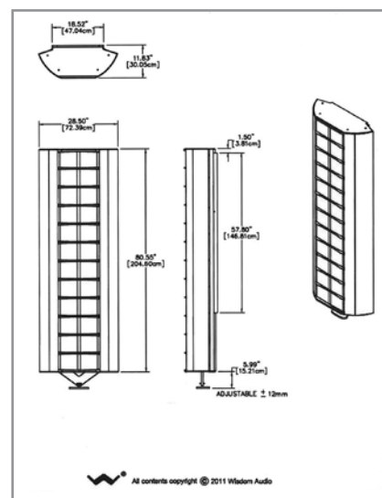
△ LS4 尺寸圖。
